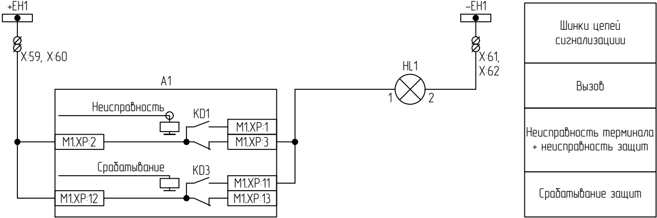
Цепи сигнализации
